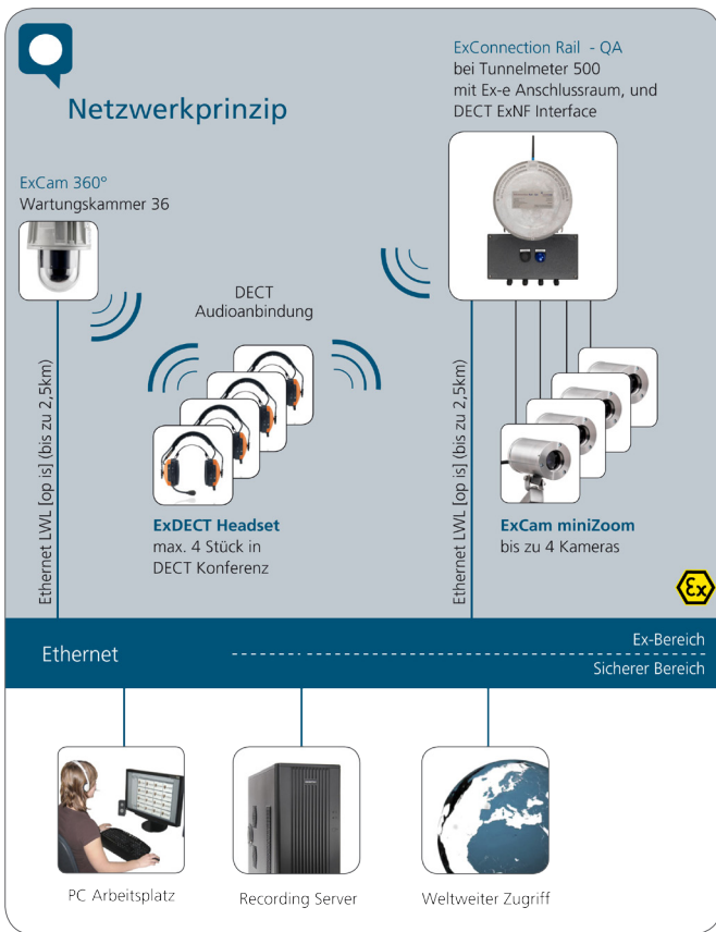
Bild 2: Netzwerkausschnitt Biomasse Deponie ABlar
